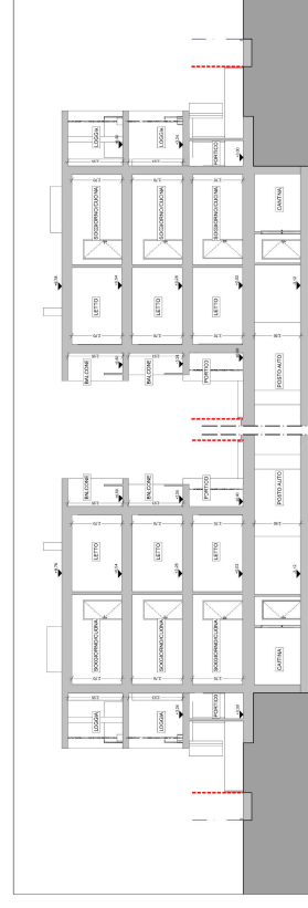
SEZIONE A-A
